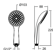
3524D1 11,70 € 99Z306239 ● Ducha de mano de ABS con 1 función. ABS hand shower with 1 function.
