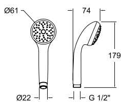
351502SC 5,90 € 99Z305273 ● Ducha de mano de ABS con 1 función. ABS hand shower with 1 function.
