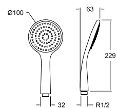
3521NL 20,90 € 241377 ● Ducha de mano de ABS con 1 función. ABS hand shower with 1 function.
