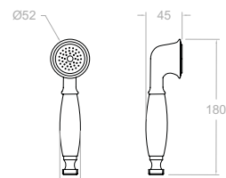
1224 28,80 € 179232 ● Ducha de mano de ABS con 1 función. ABS hand shower with 1 function.
